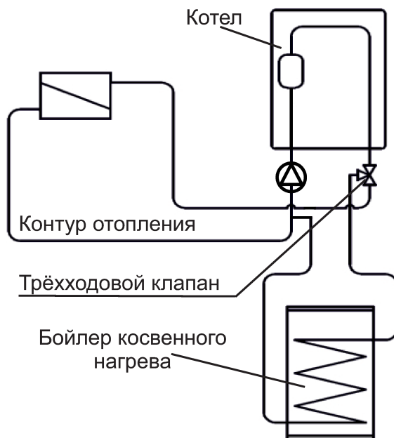
Рисунок 25. Гидравлическое подключение комплекта ГВС EVAN AQUA.
