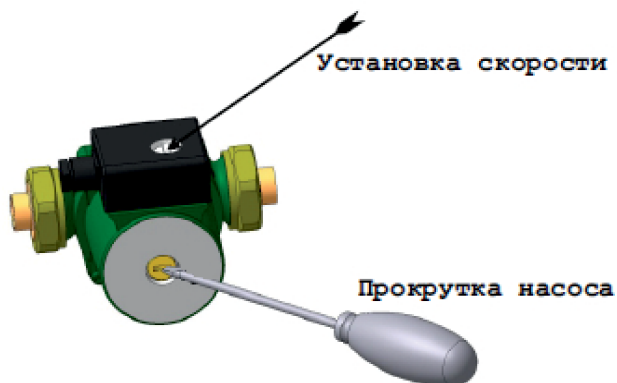
Рисунок 36. Схема обслуживания насоса.
