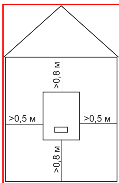
Рисунок 12. Схема установки прибора.
