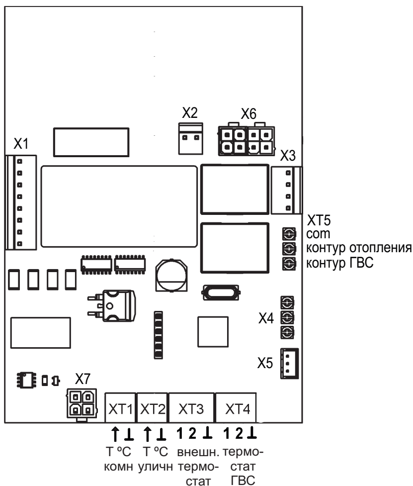
Рисунок 5. Подключение к разъёмам на плате.
