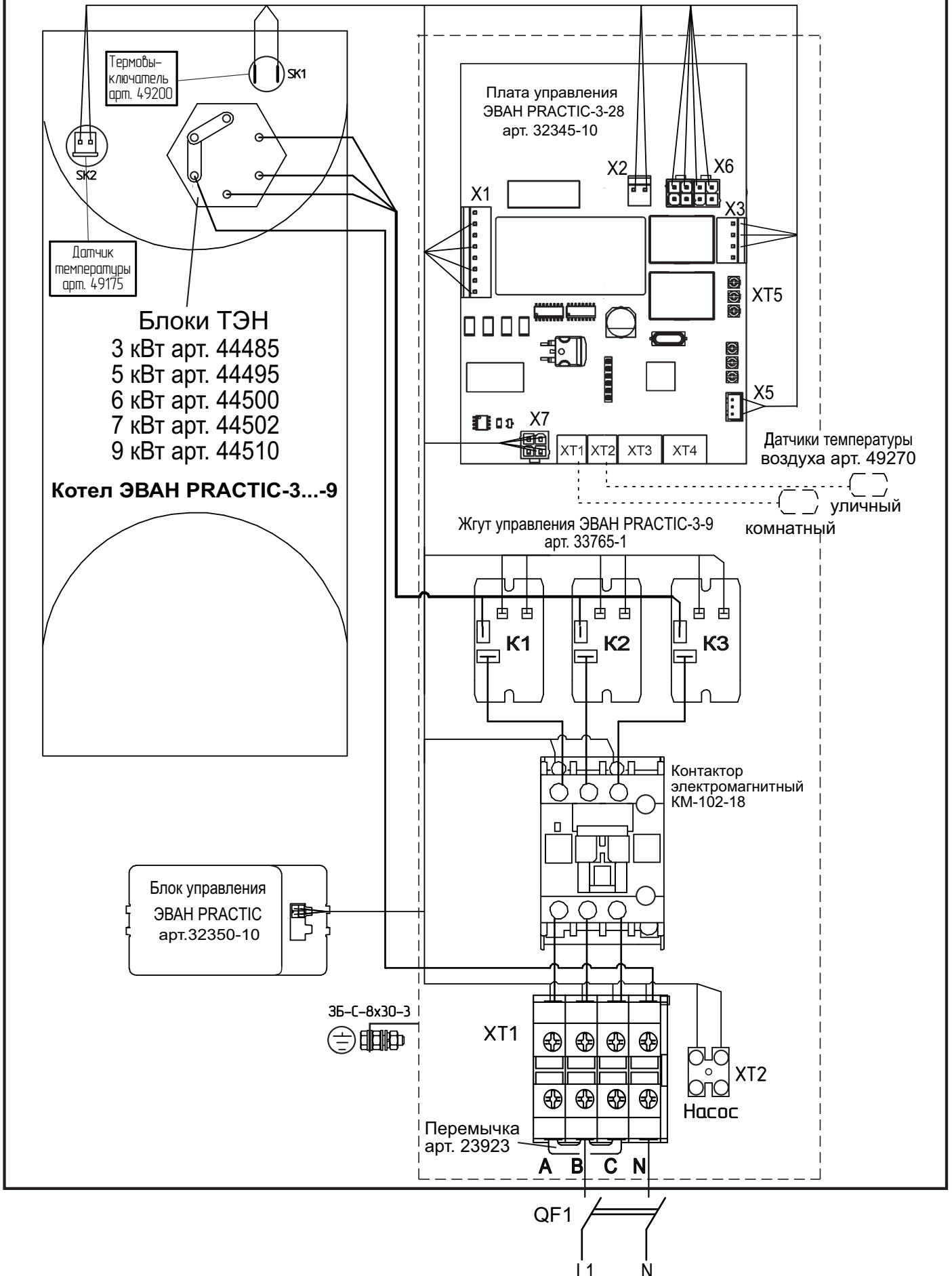
Рисунок 18. Схема подключения ЭВАН PRACTIC-3...-9 к сети 220В.
