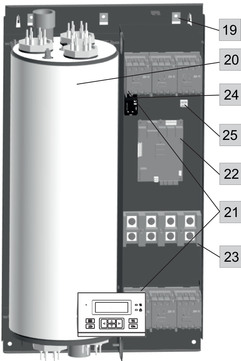
Рисунок 4. Прибор ЭВАН PRACTIC -72 ... -120 со снятым кожухом.
