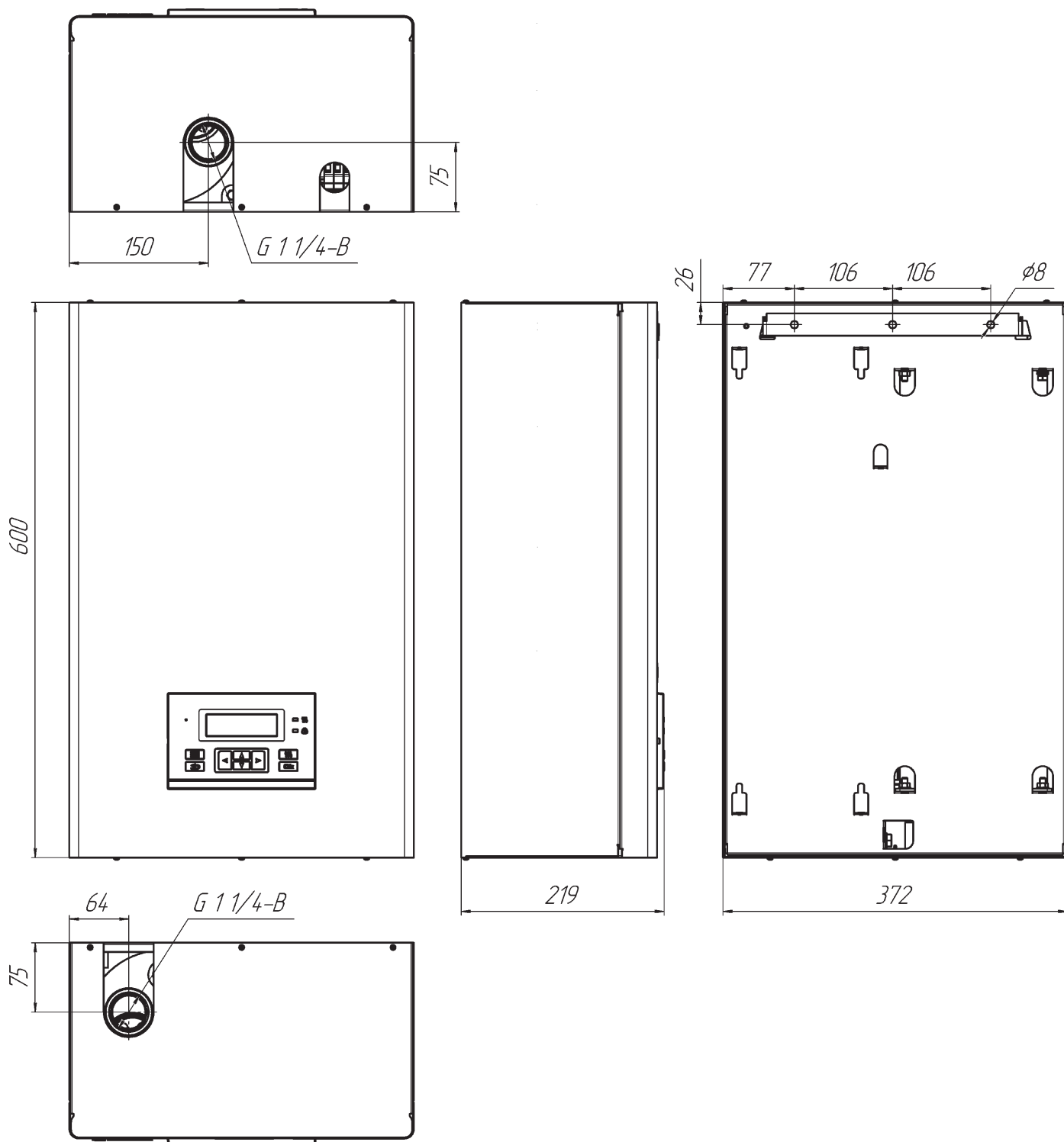
Рисунок 16. Габаритные и присоединительные размеры прибора ЭВАН PRACTIC -3 ... -28
