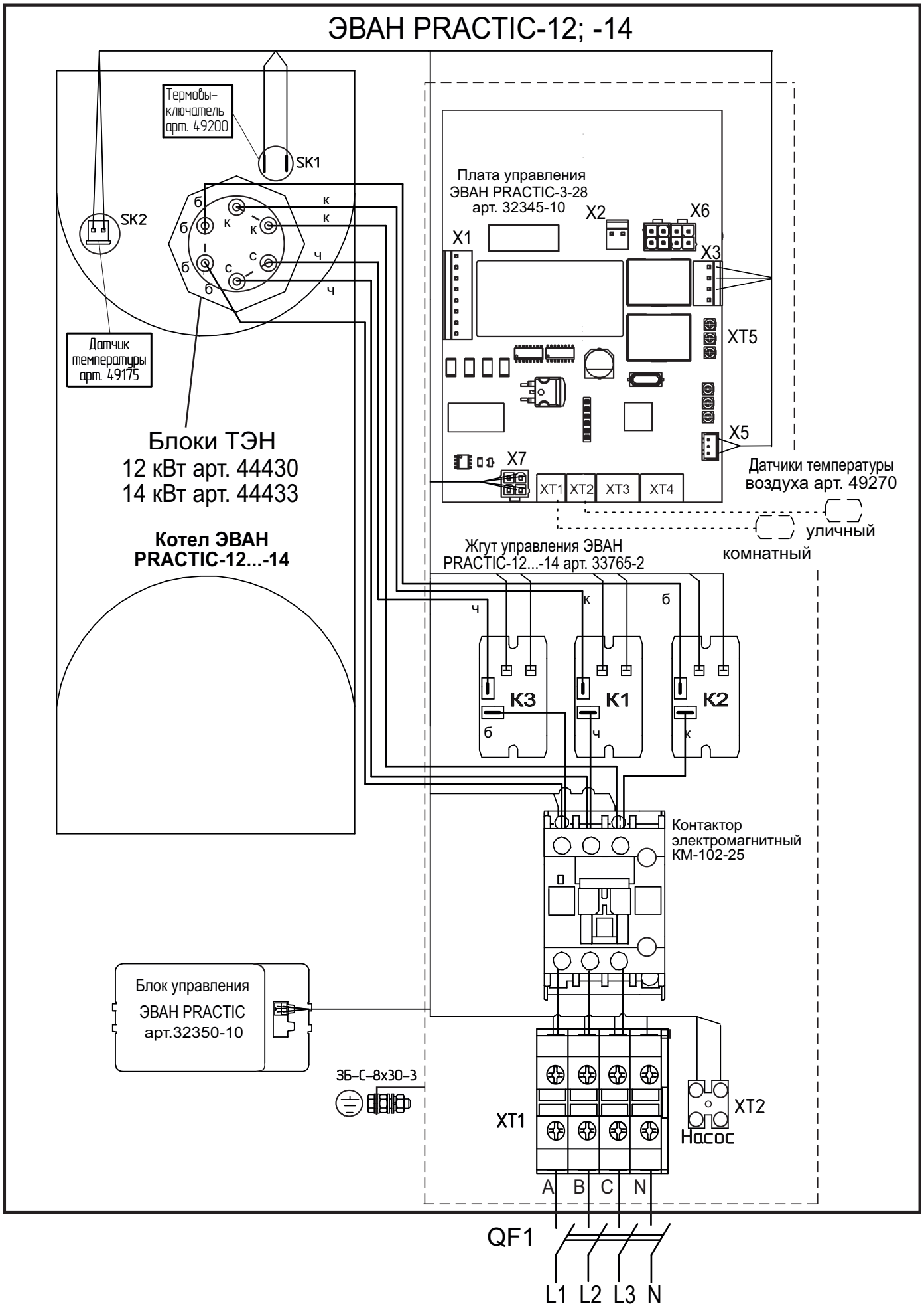
Рисунок 20. Схема подключения ЭВАН PRACTIC-12; -14.
