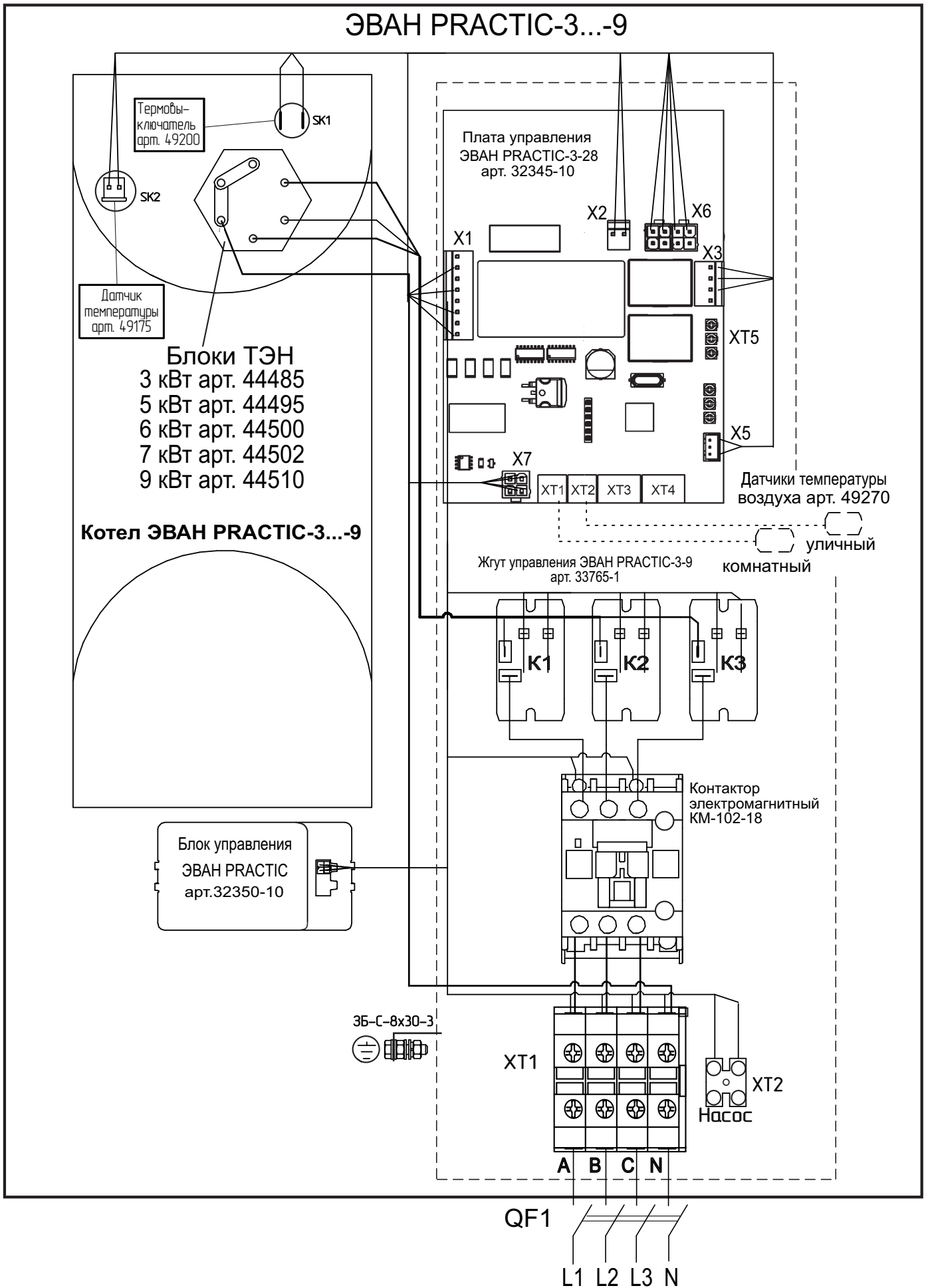
Рисунок 19. Схема подключения ЭВАН PRACTIC-3...-9 к сети 380В.
