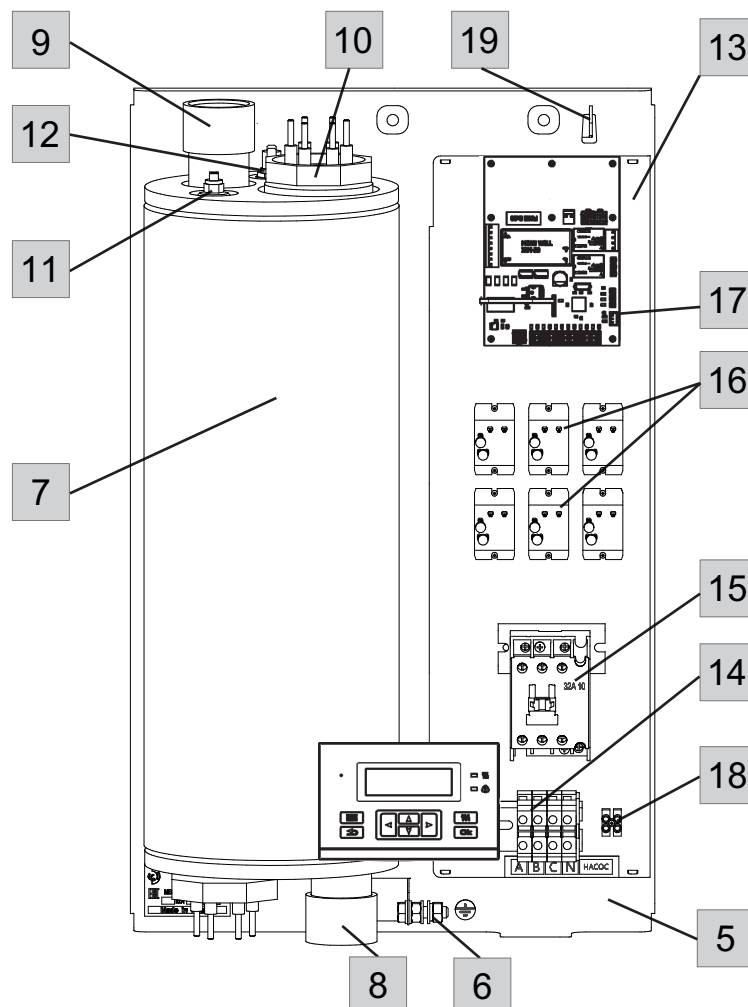
Рисунок 3. Прибор ЭВАН PRACTIC - 18 ... -28 со снятым кожухом.
