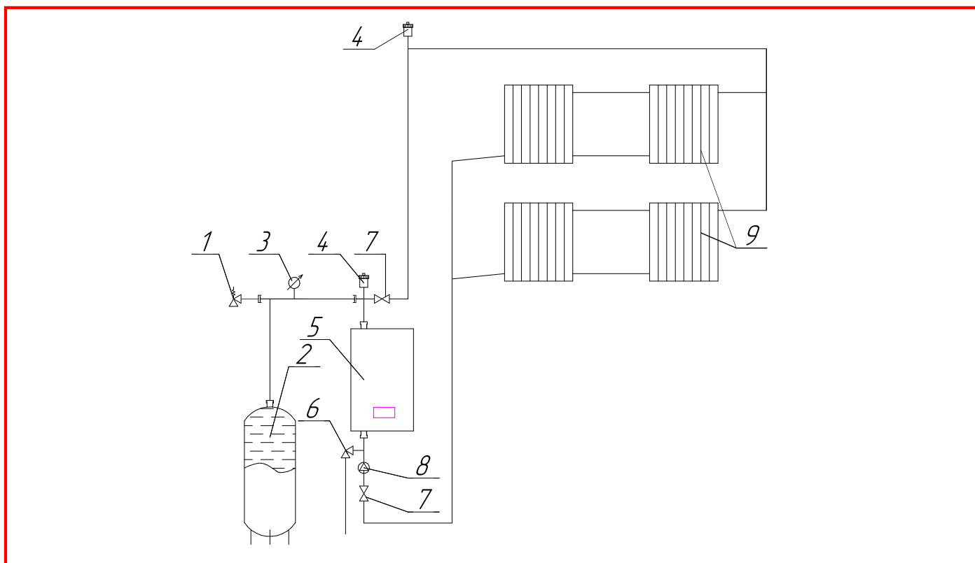
Рисунок 13. Гидравлическая схема отопительной системы 1 - Клапан предохранительный; 2 - Экспанзомат; 3 - Манометр; 4 - Воздухоотводчик автоматический; 5 - Прибор; 6 - Кран сливной; 7 - Краны шаровые; 8 - Насос циркуляционный; 9 - Радиаторы
