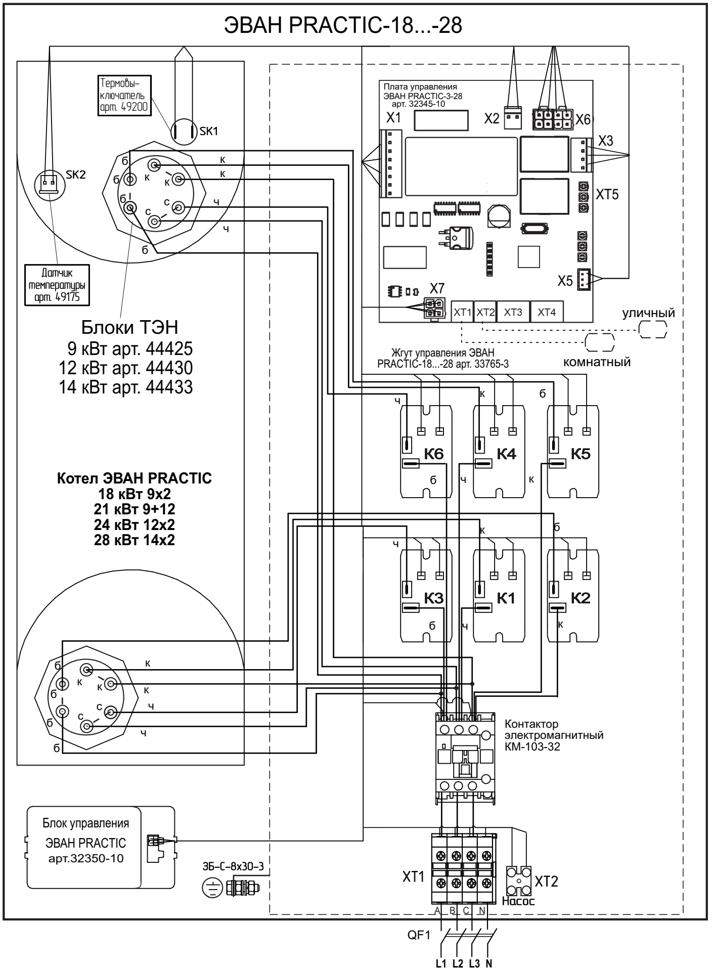
Рисунок 21. Схема подключения ЭВАН PRACTIC-18...-28.
