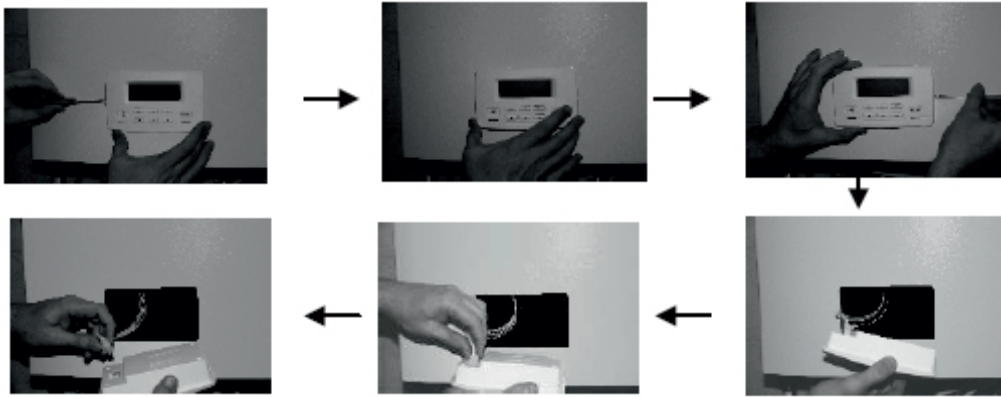
Рисунок 2. Порядок извлечения блока управления.
