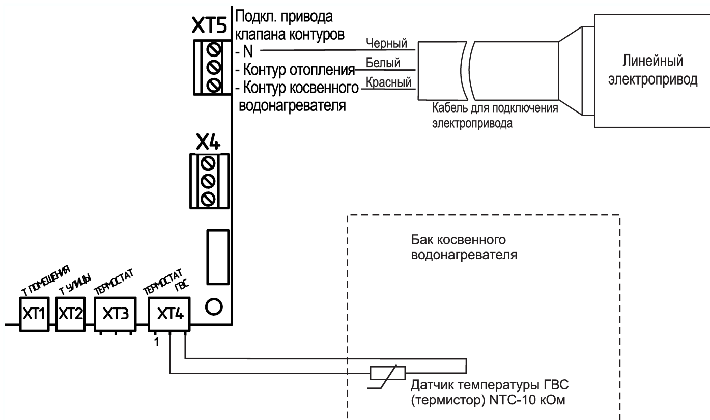
Рисунок 24. Электрическое подключение комплекта ГВС EVAN AQUA.
