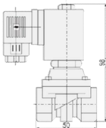
Рисунок 1. Эскиз
